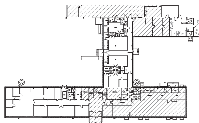
ENTRÉPLAN
