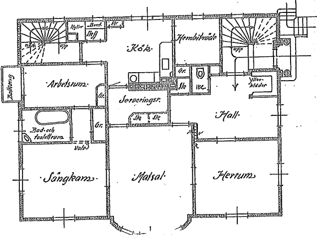
Plan av 1 te & 2 de Vån.
