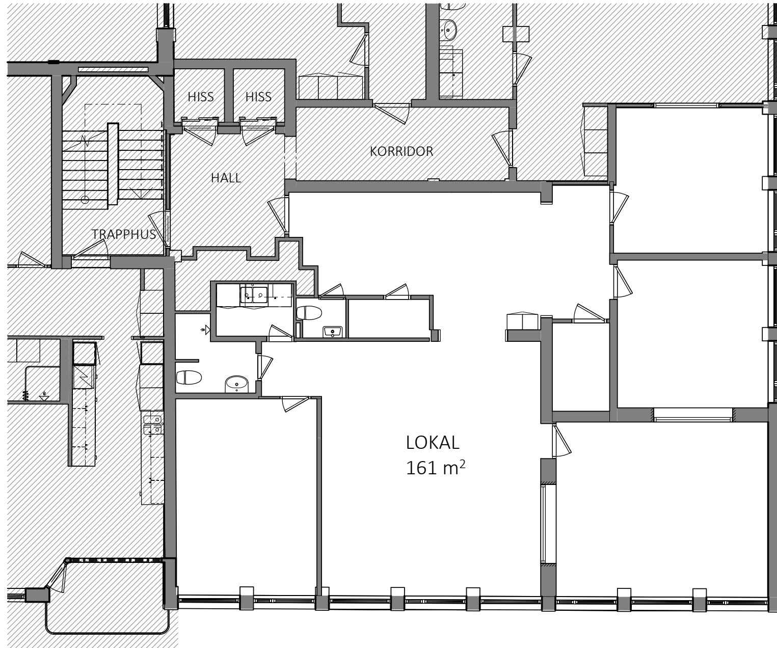
PLAN 14 - VÅNING 4
