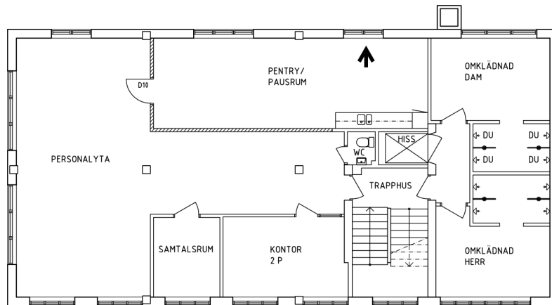
PLAN 3, VÅNING 1 TR.
