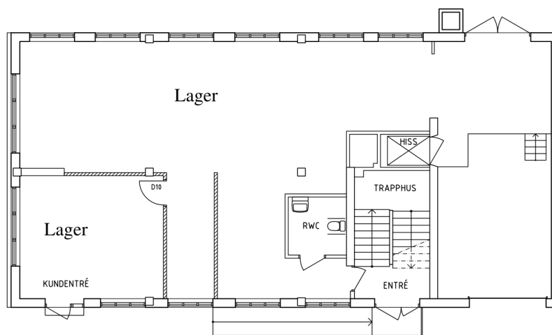
PLAN 2, ENTRÉVÅNING
