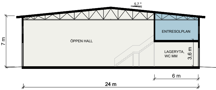
PRINCIPSEKTION A 1:300
