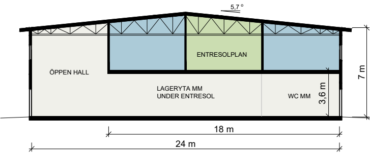
PRINCIPSEKTION A 1:300
