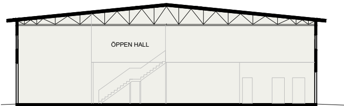
PRINCIPSEKTION B 1:300
