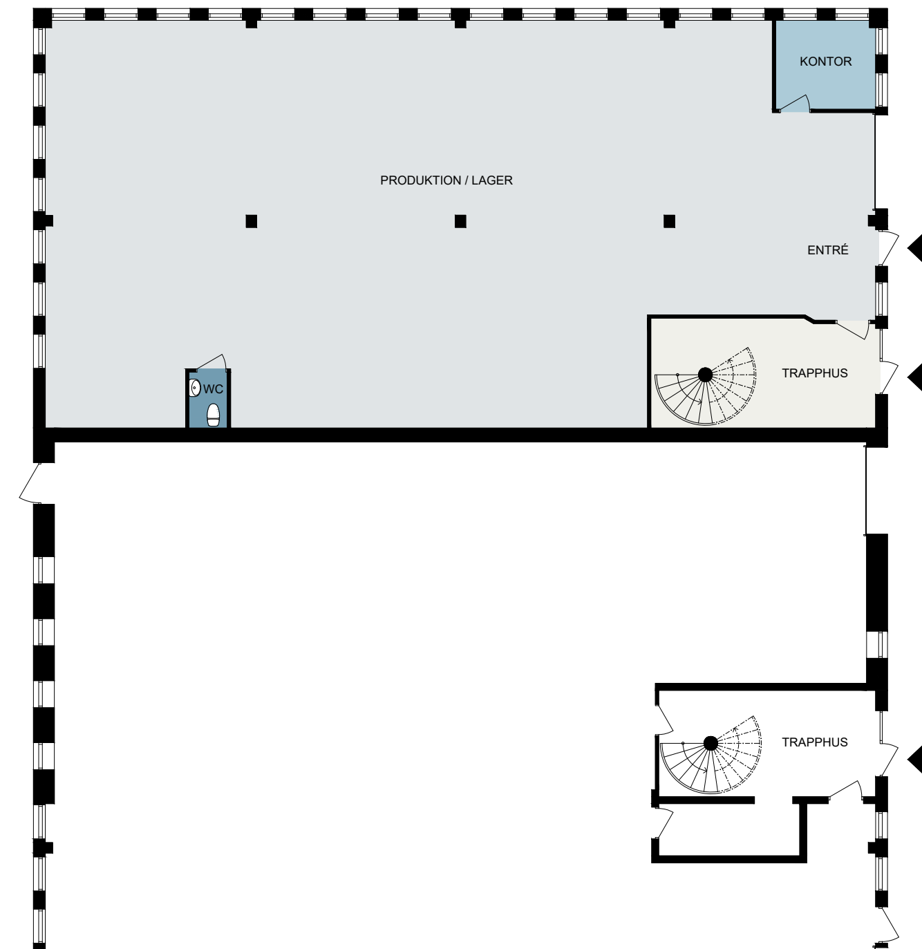
PLAN 1, ENTRÉVÅNING
