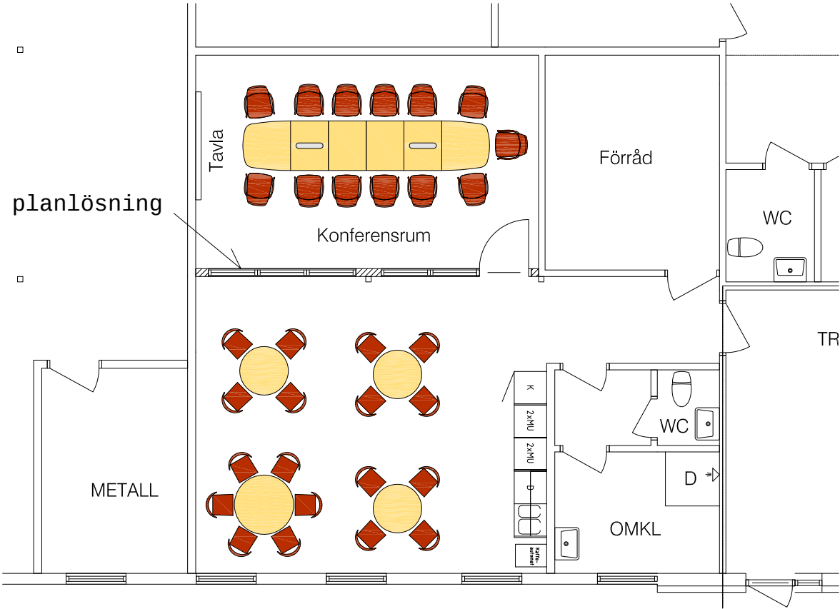
Delplan 0 1:50
