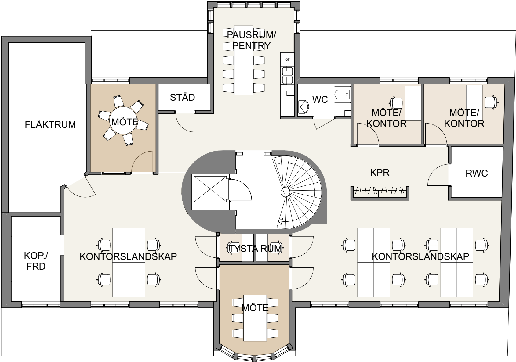
PLAN FYRA TRAPPOR Skala 1:100 (A3)
