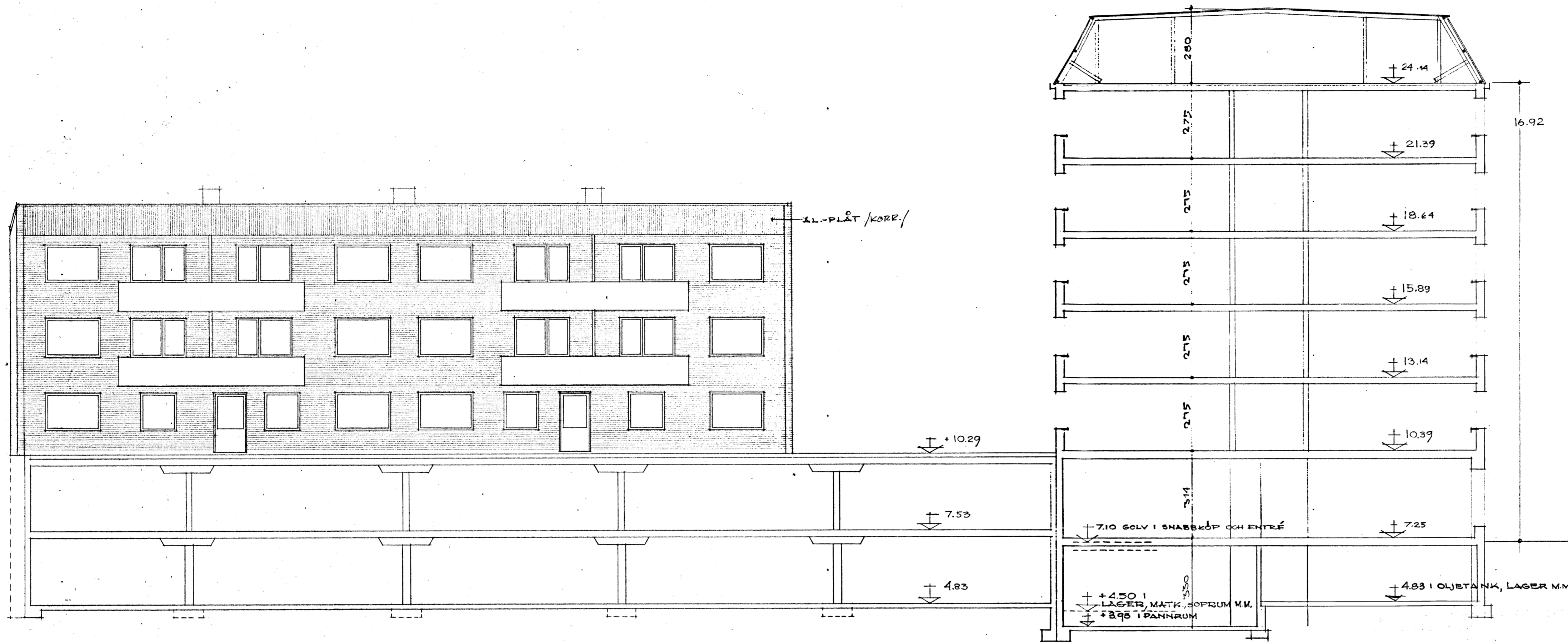
SEKTION B-B : FASAD MOT SÖDER (HUSA)
