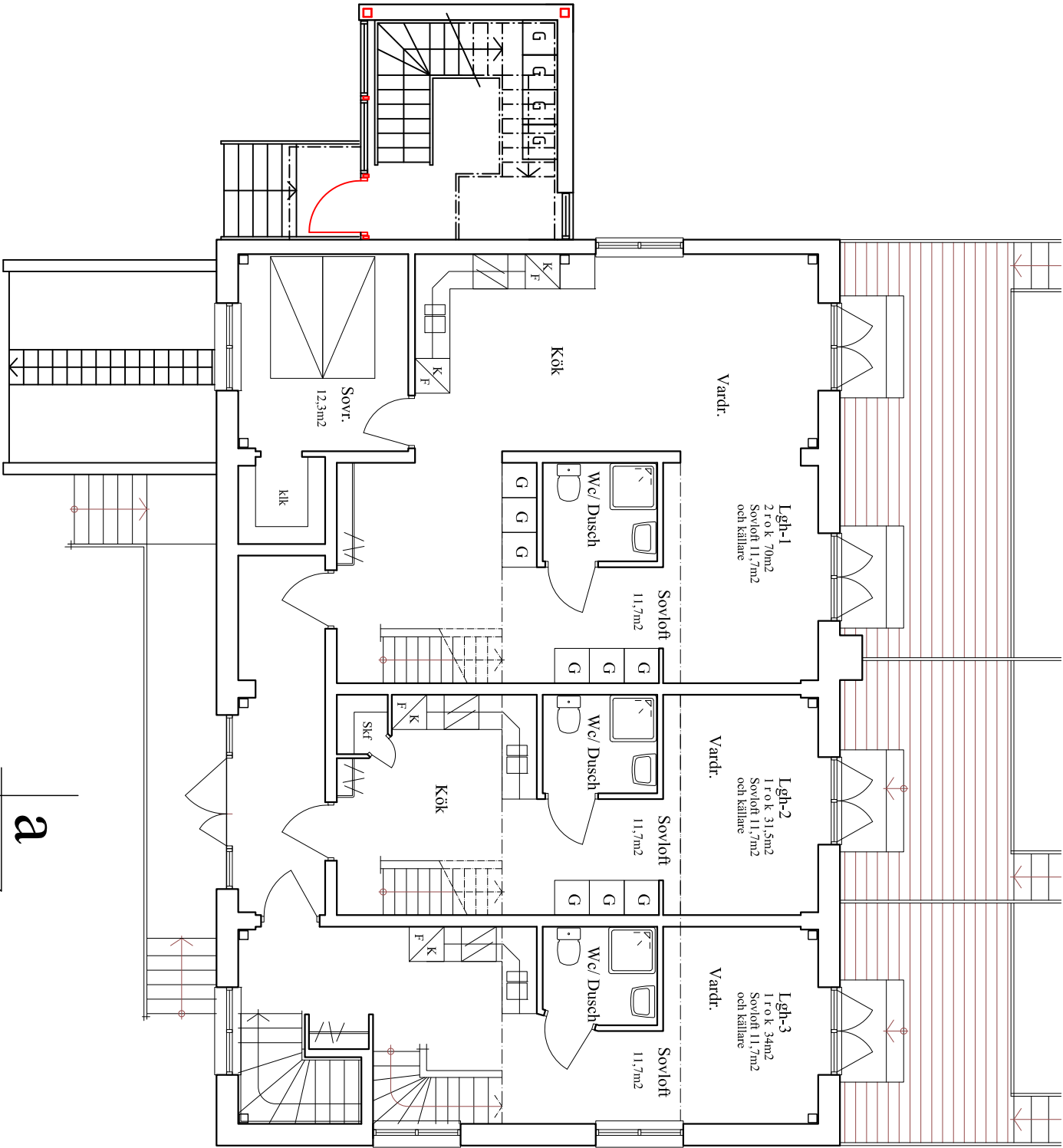
Plan vån-1, skala 1:100
