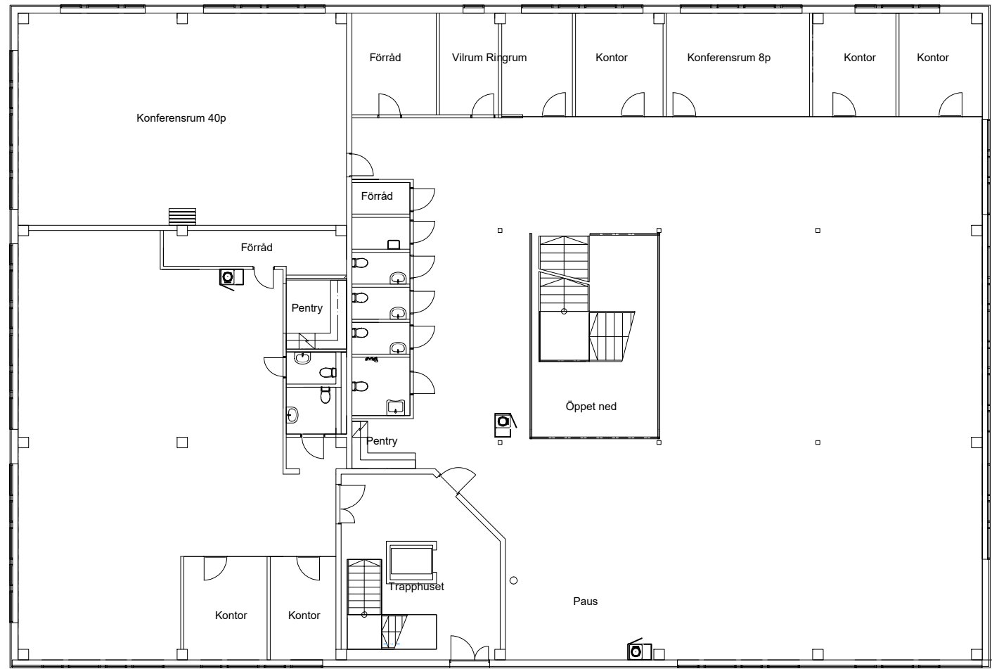
Övervåning 1:100
