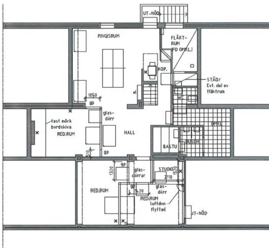
PLAN 1 - KÄLLAREN LOA 131 m 2
