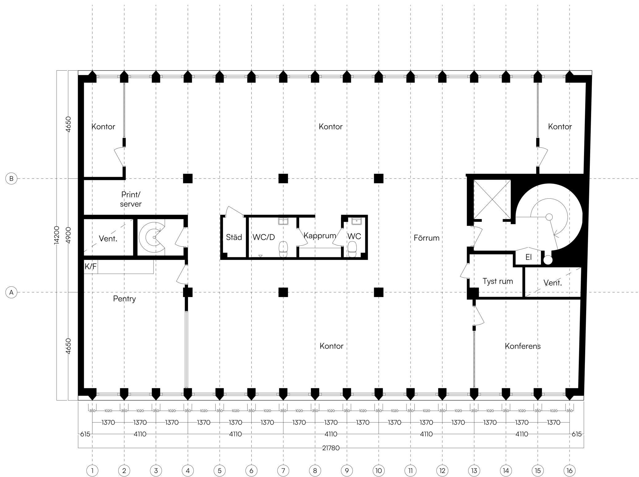
KUNGSGATAN 71, PLAN 4
