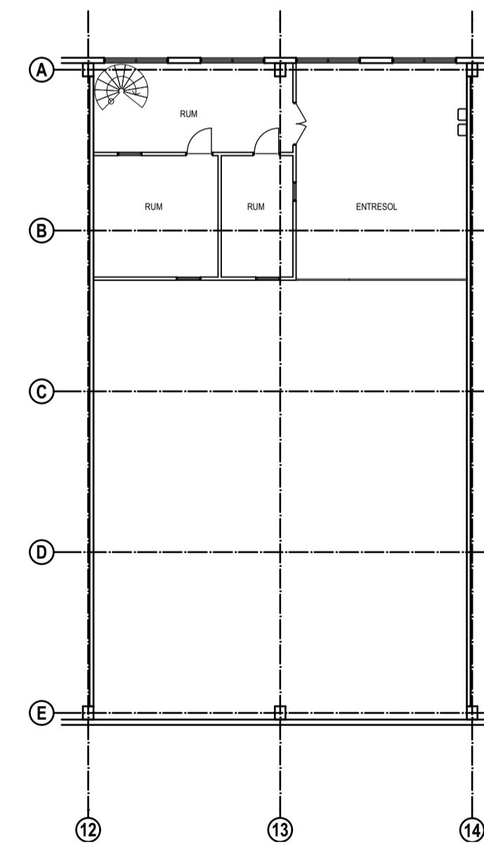
ENTRESOL 1:200
