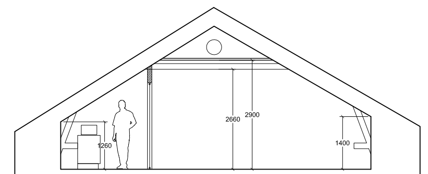
SEKTION B-B
