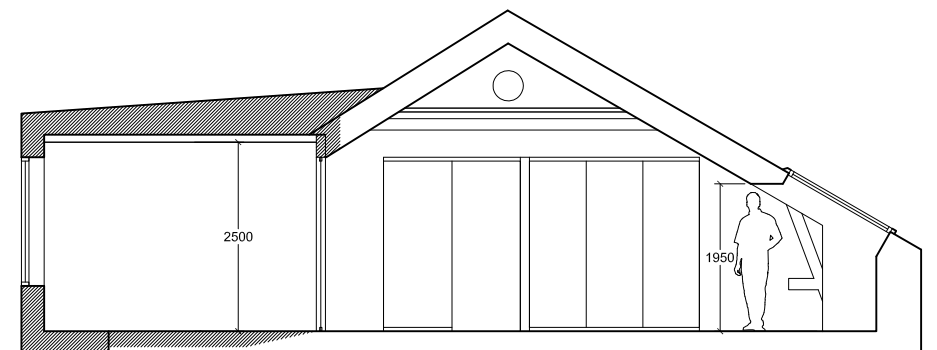
SEKTION A-A
