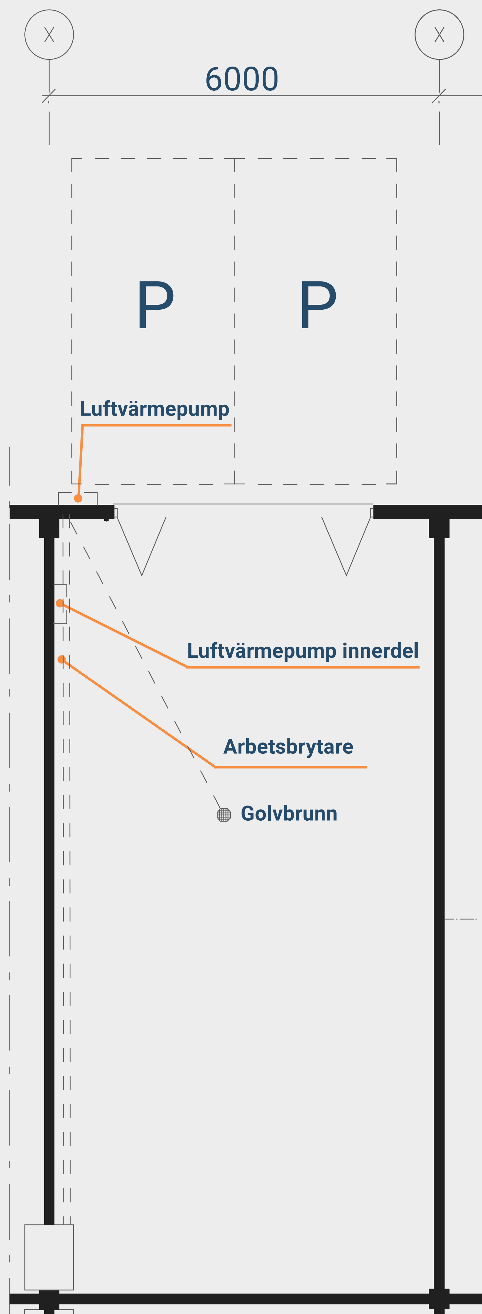
PLAN BOTTENVÅNING
