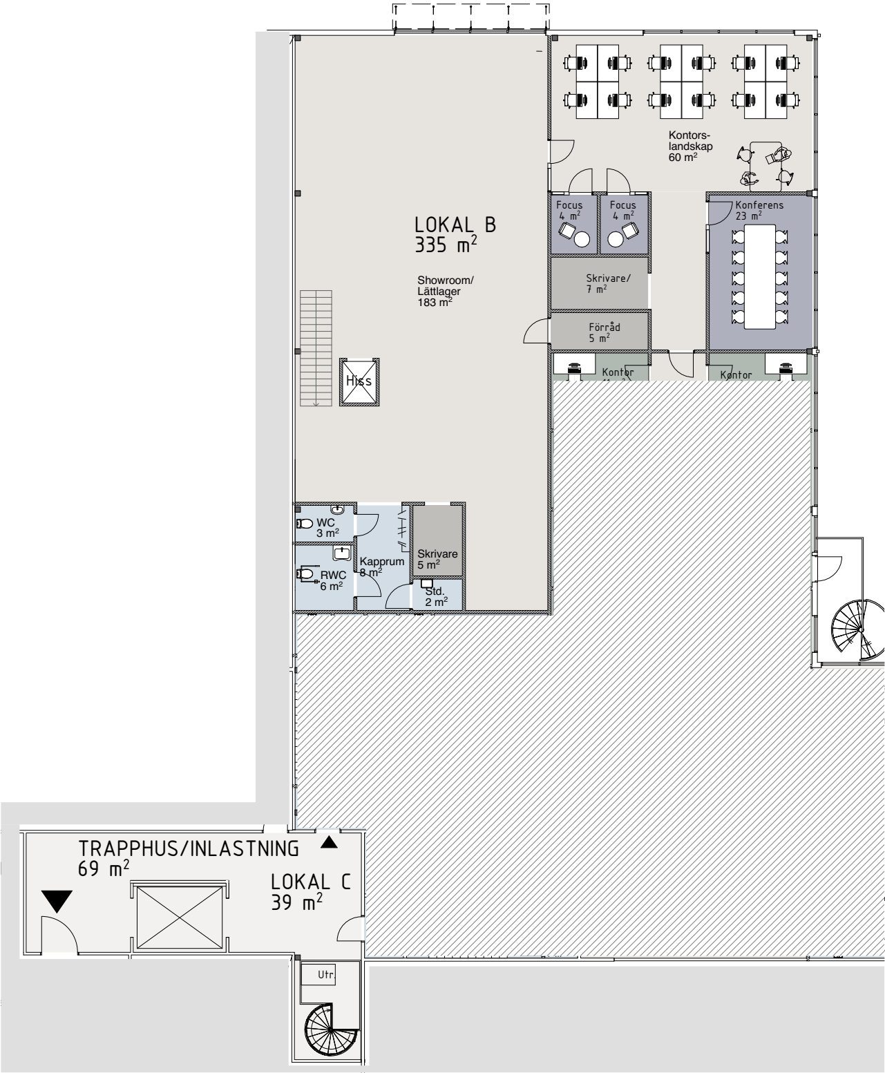
Plan 1, Entréplan 1:200
