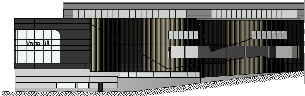
Fasad mot Öster 1:500
