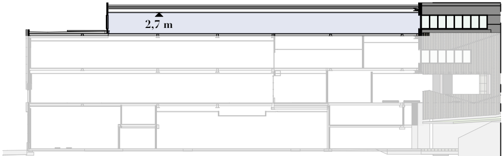
Sektion 1:500
