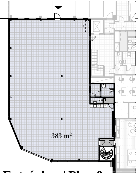
Entréplan / Plan 0
