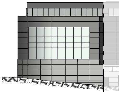
Fasad mot Söder 1:400
