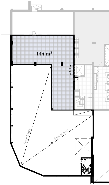
Plan - 1, Entrésol
