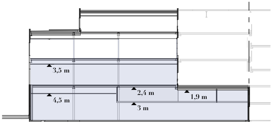
Sektion 1:400
