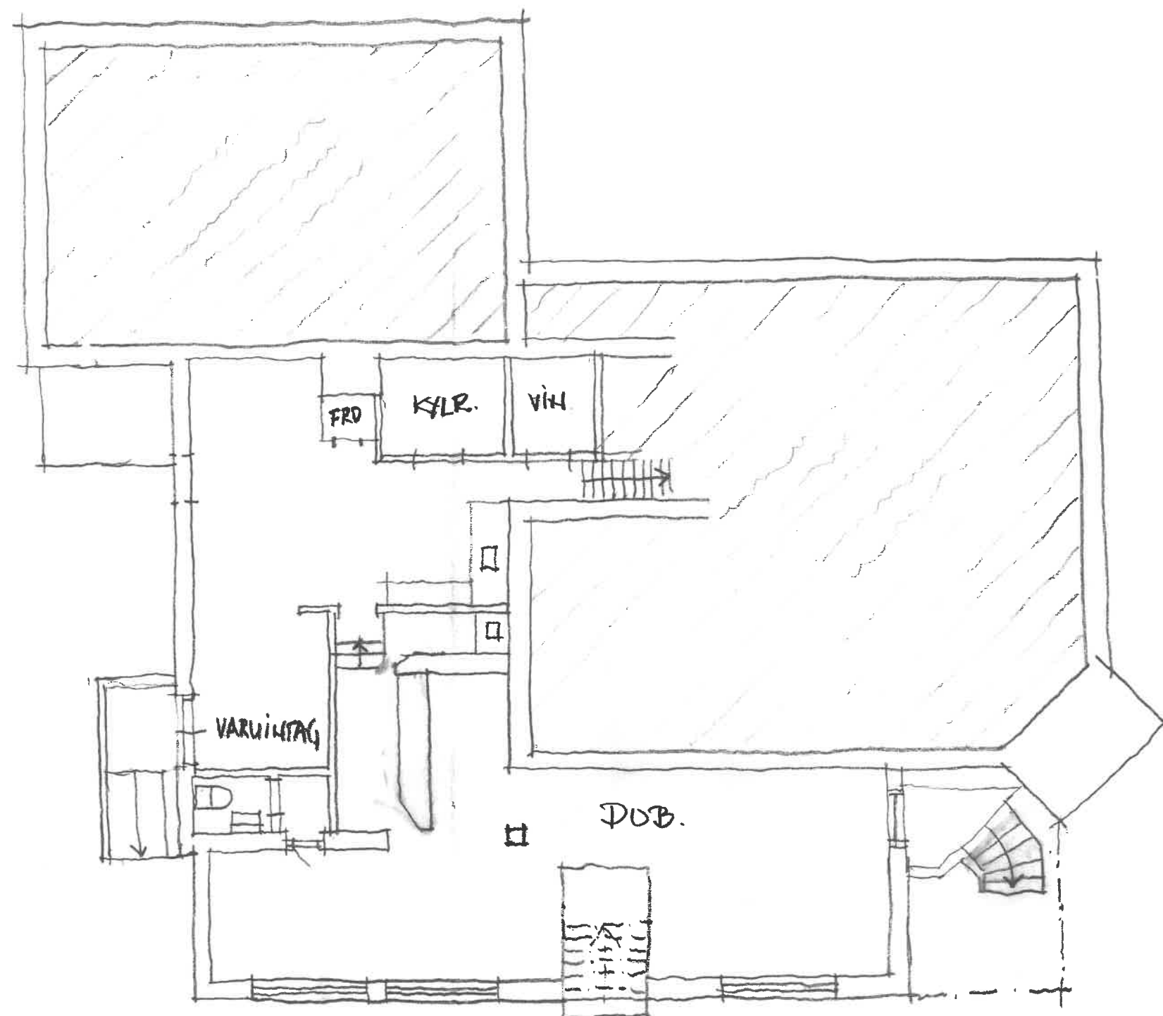
PRINCIPSSKISS KÄLLARE FLUNDRA 1:80
