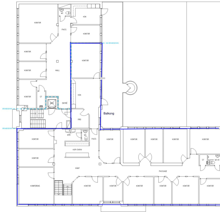
PLAN 2, VÄNING 1 TR
