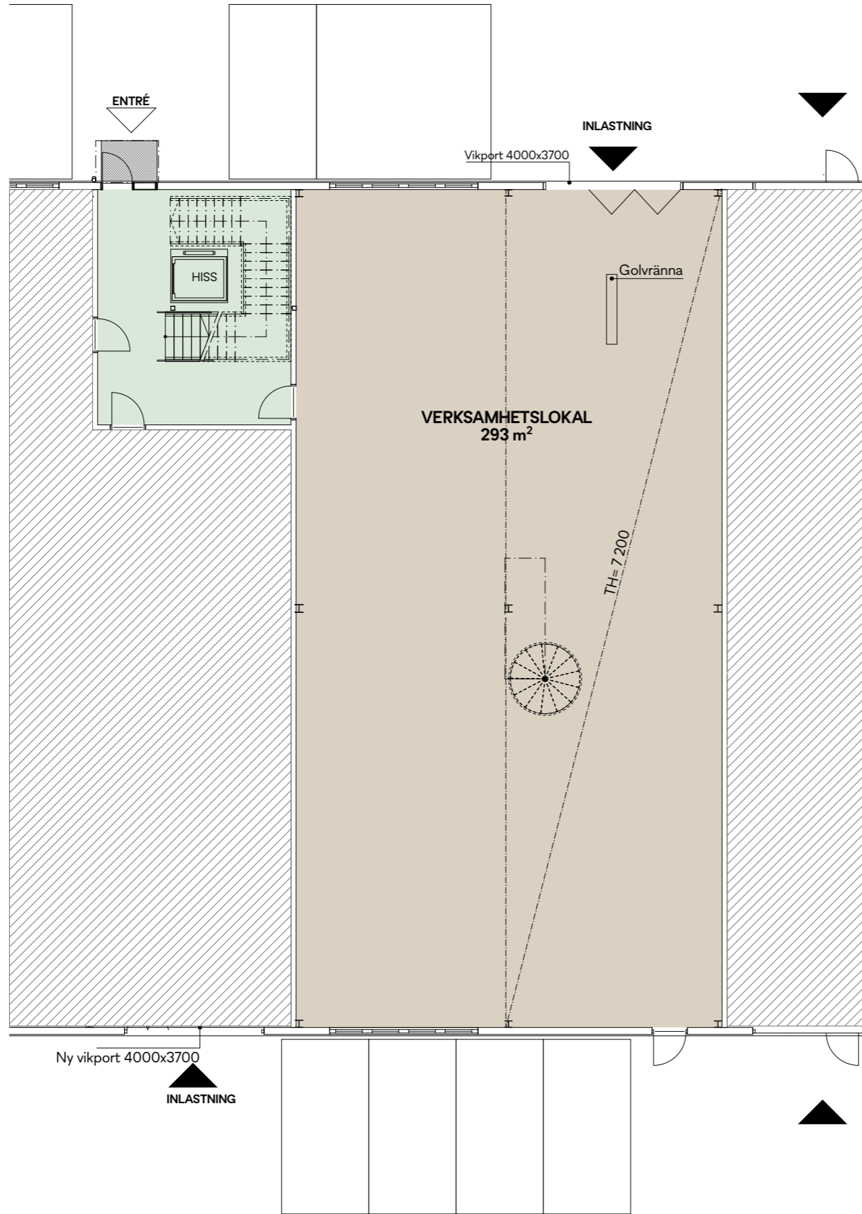
Plan 1 1:150
