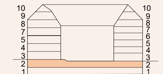
Sektion
