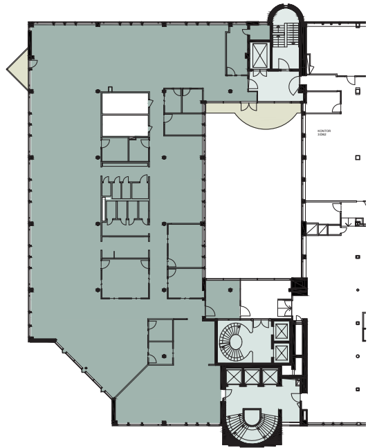
PLAN 6 (VÅN 3)
