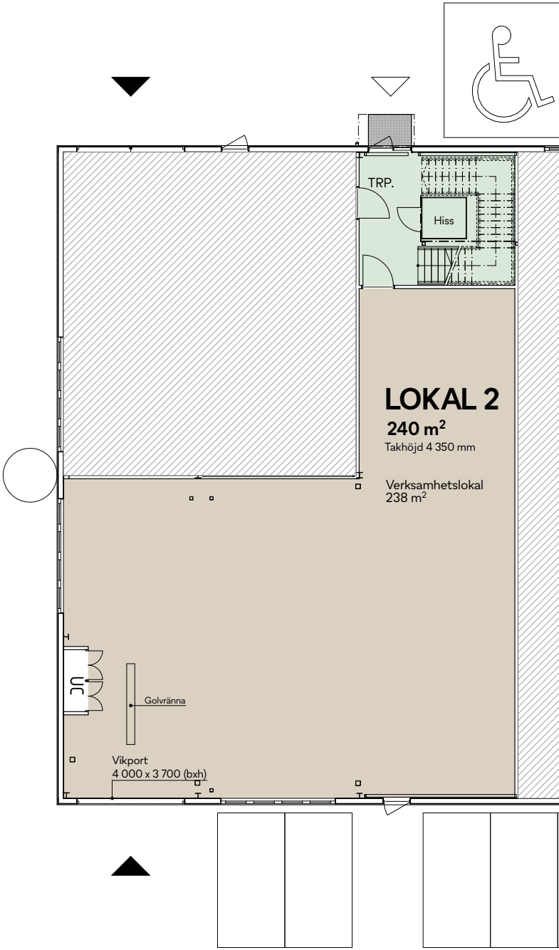
Plan 1, Entréplan 1:200
