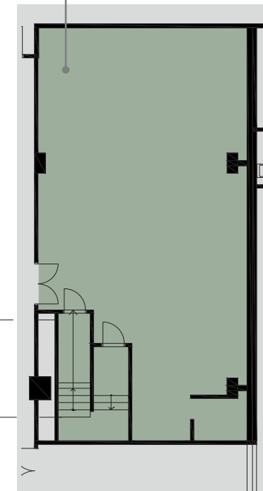
Plan -1.
