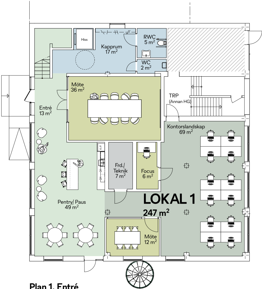
Plan 1, Entré 1:150
