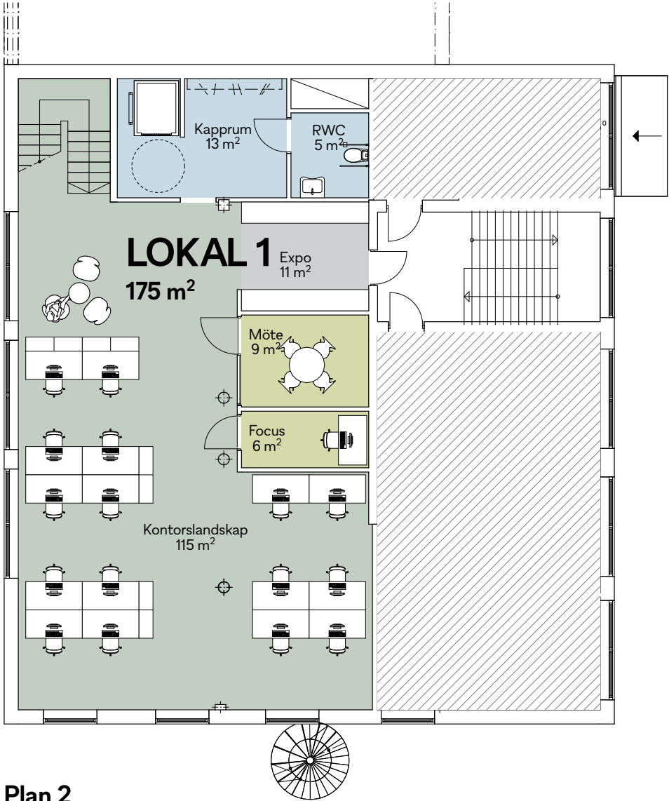
Plan 2 1:150
