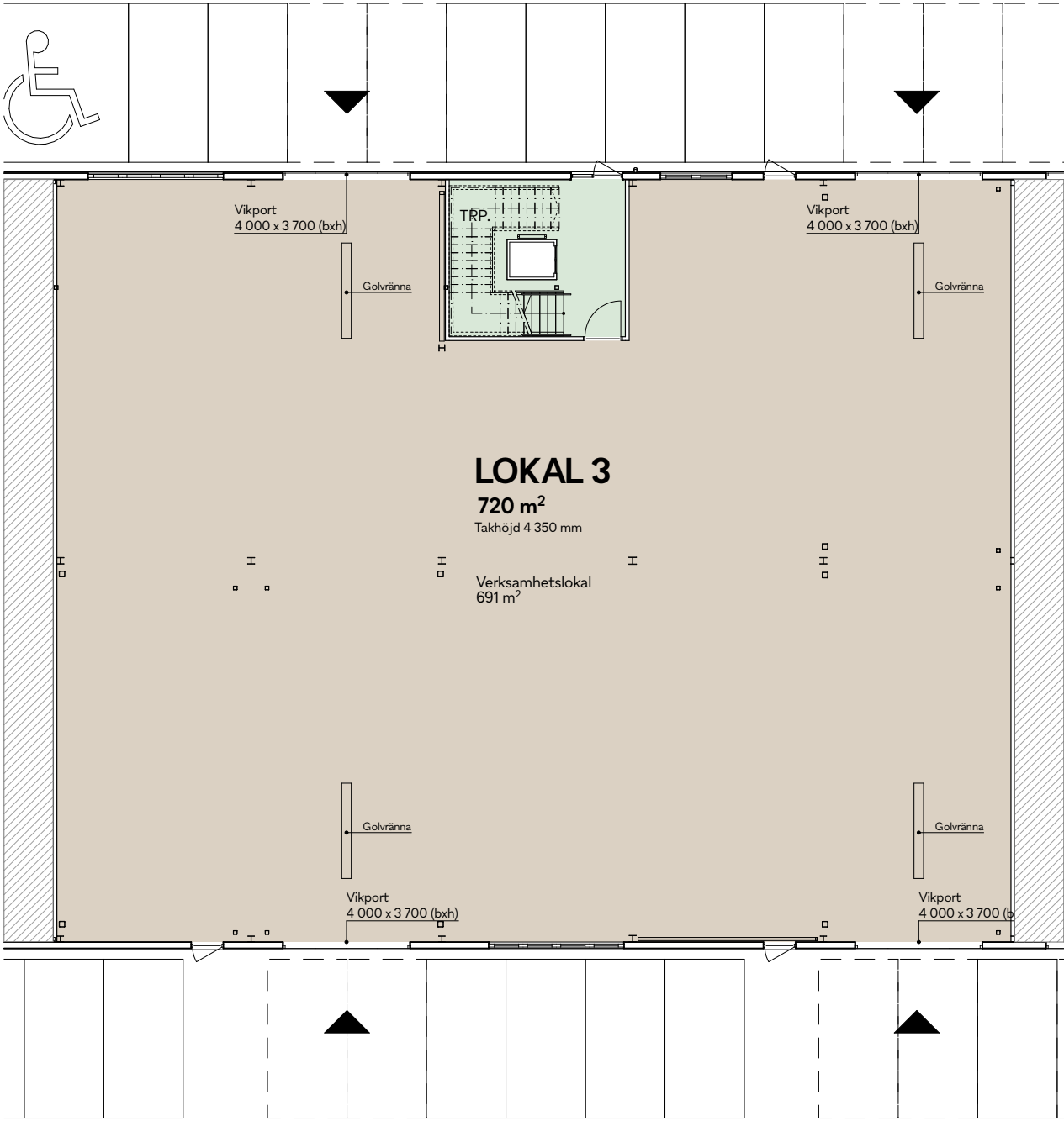
Plan 1, Entréplan 1:200
