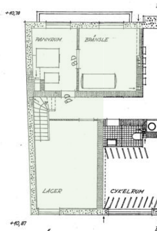
Källarplan
