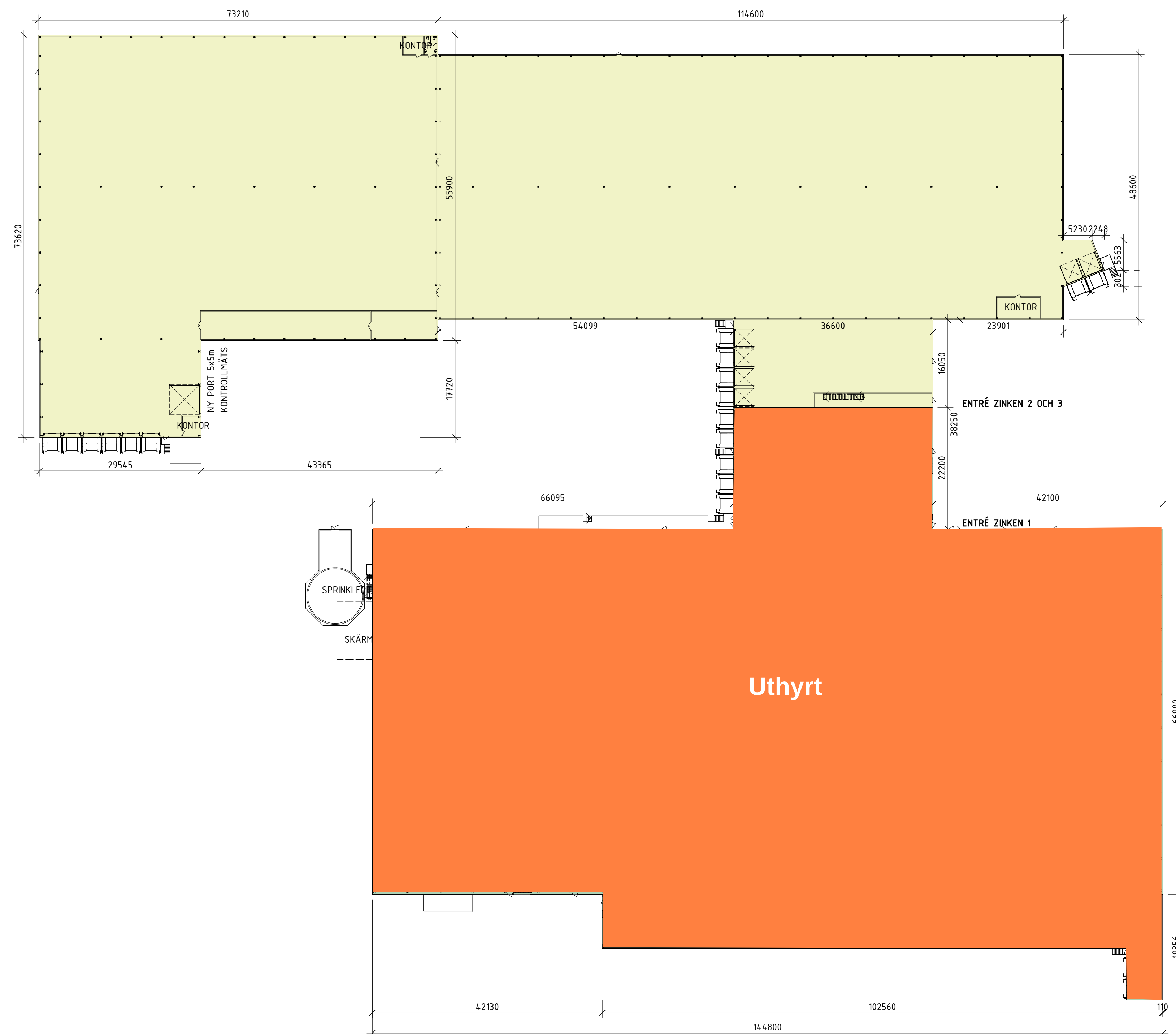
Plan 0, +3,72, fastighetsdelning 1 : 500
