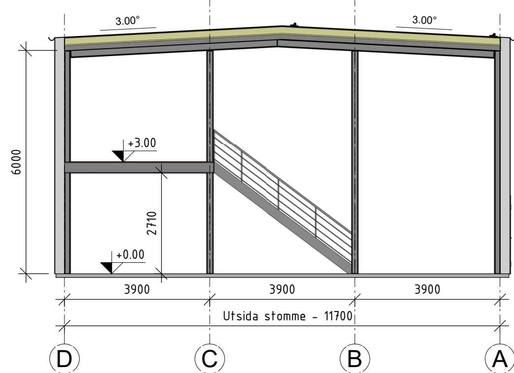
2 A1-E1 A-A 1 : 100
