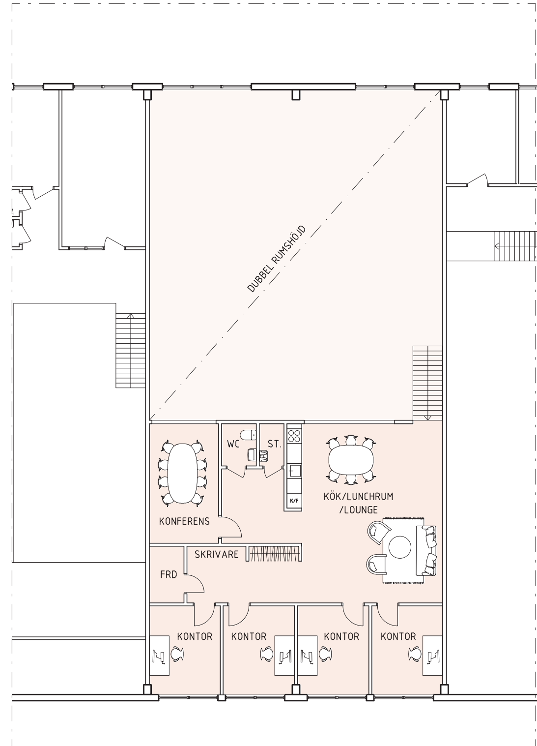
Övre plan 129 kvm LOA
