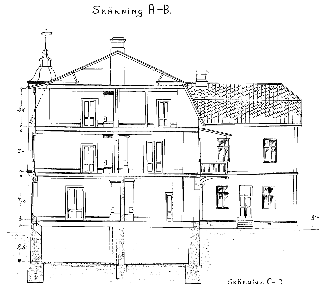
SKÄRNING A-B.
