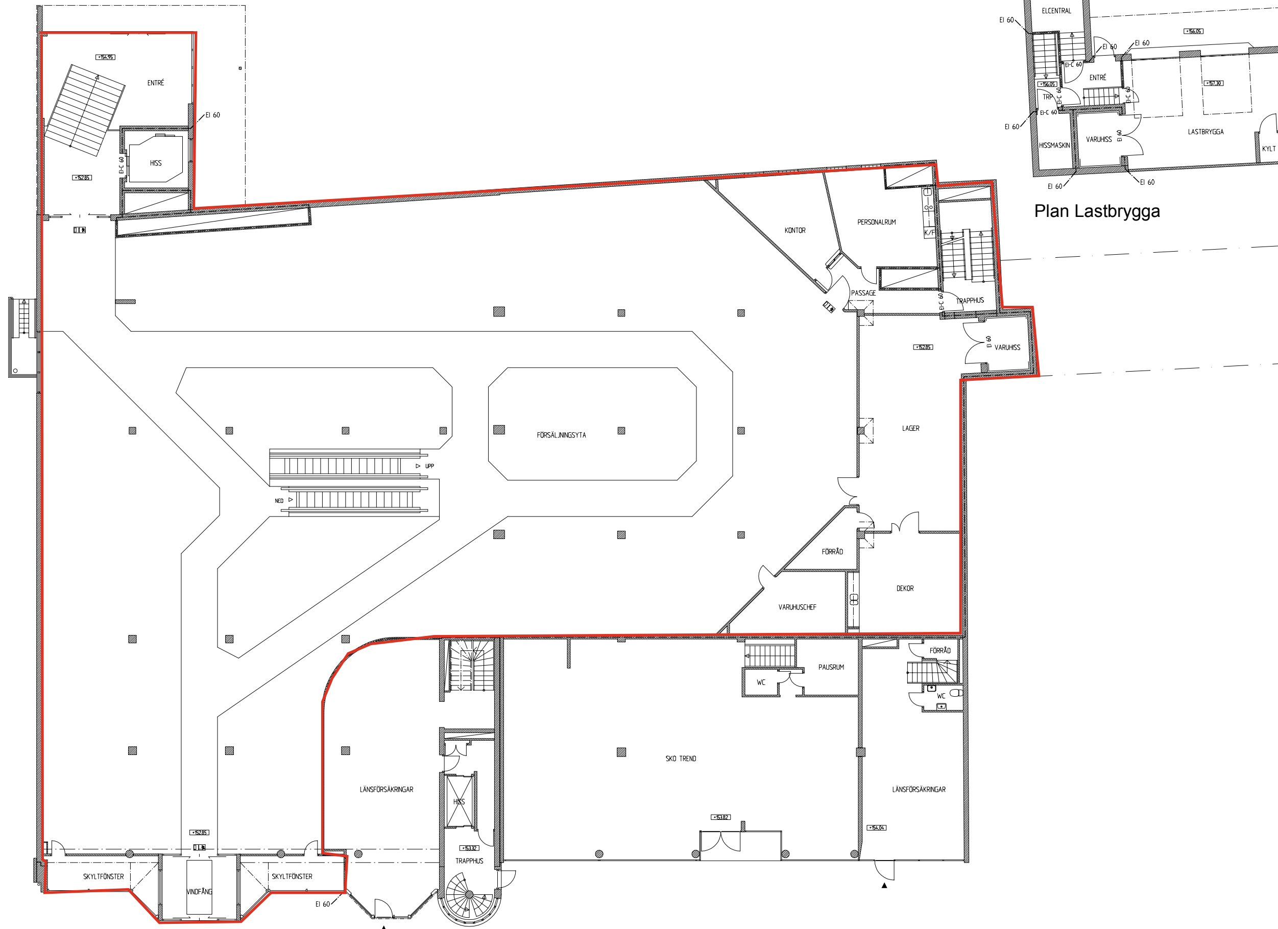
Plan Bottenvåning Skala 1:100
