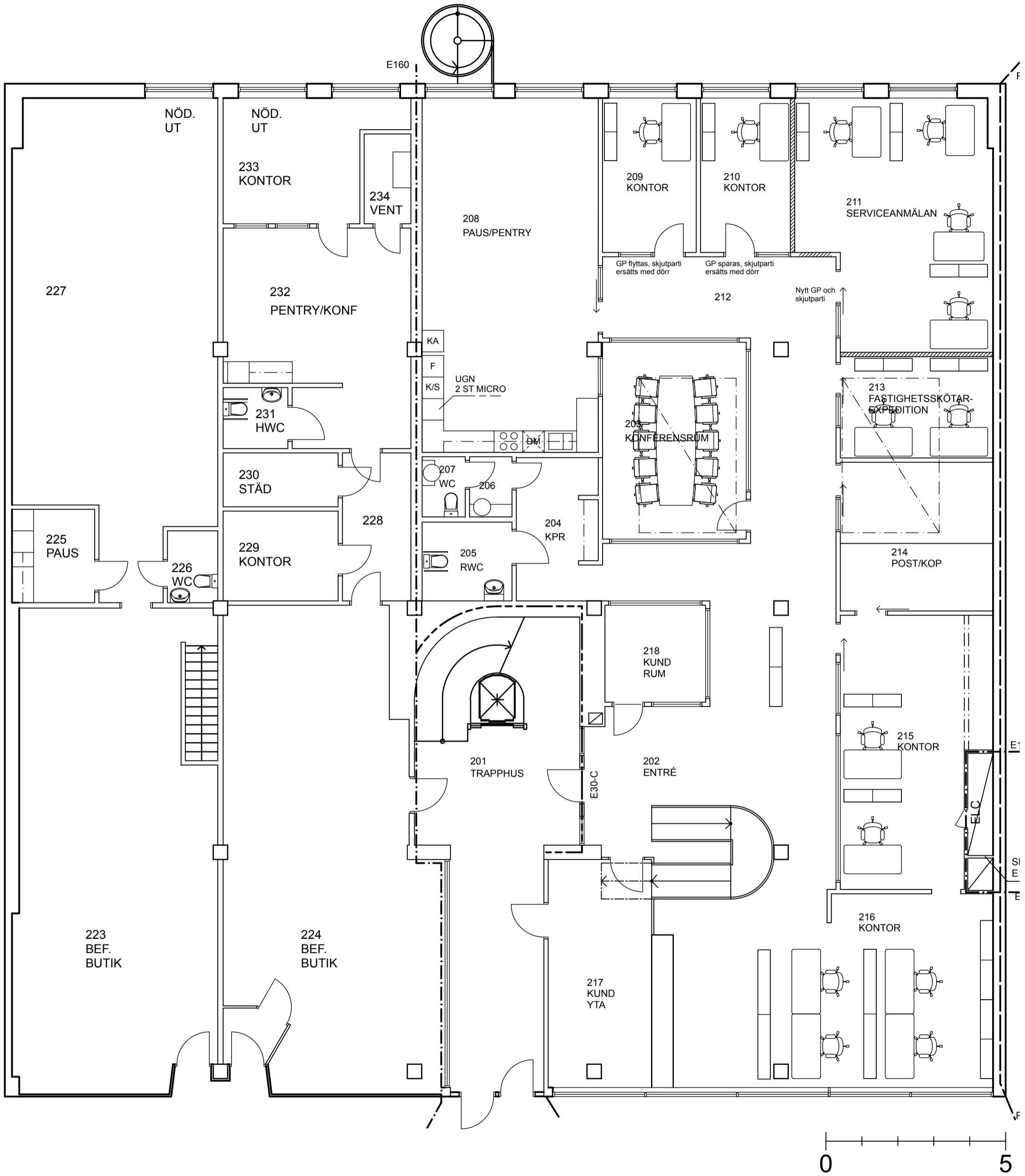
Kv Markattan 12 - Norrköping - Plan 2 - Skiss för Heimstaden Skala 1:100
