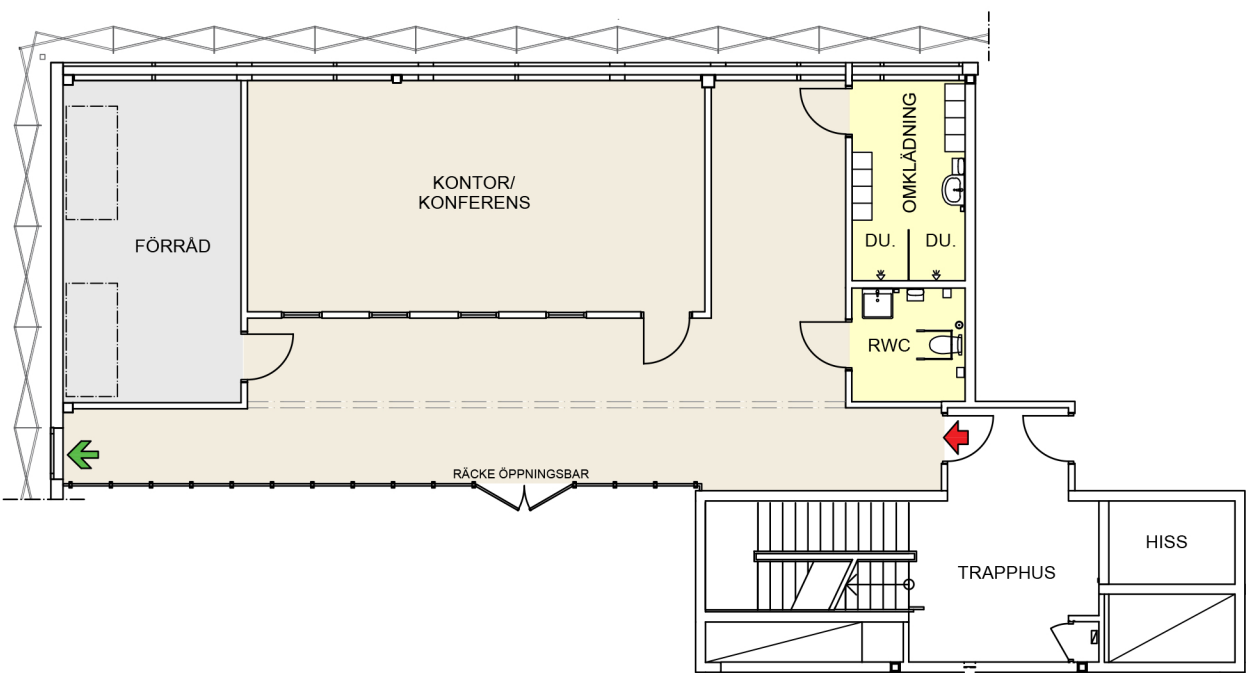
Entrésolplan Kontor
