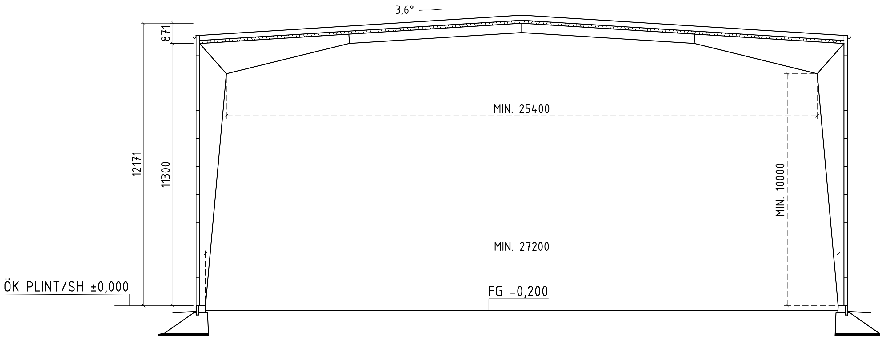
SEKTION A-A 1:100
