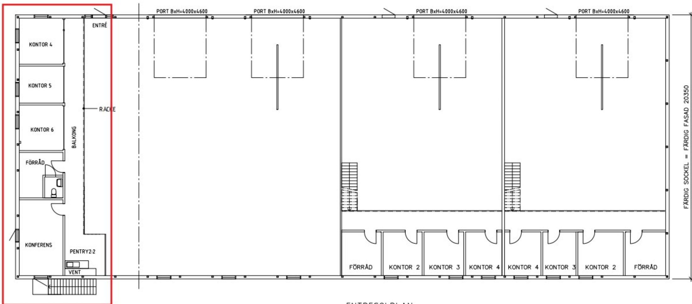
ENTRESOLPLAN 1:100
