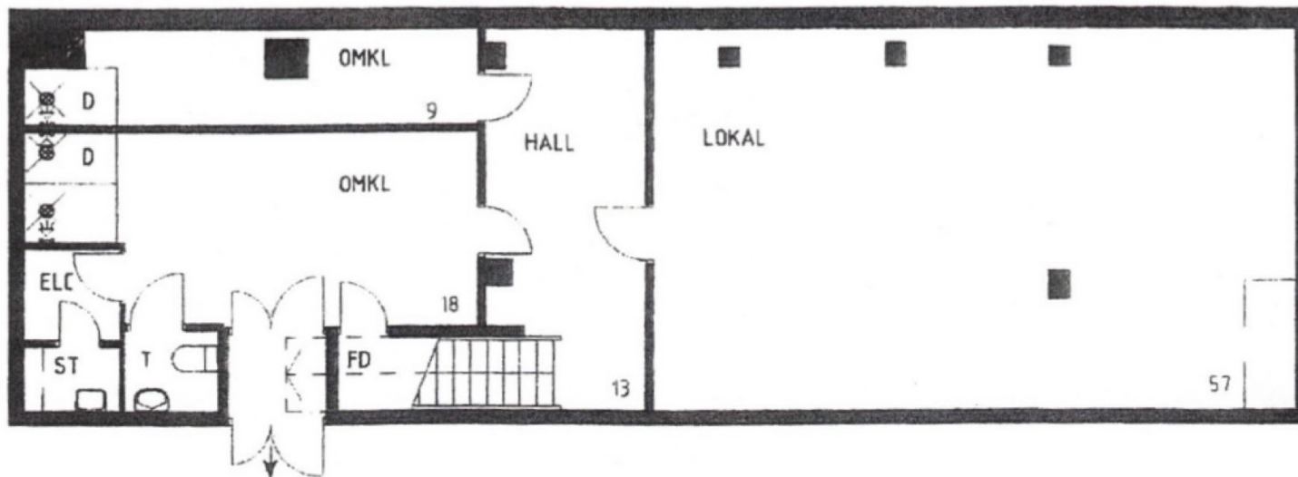
KÄLLARVÅNING 113 m 2
