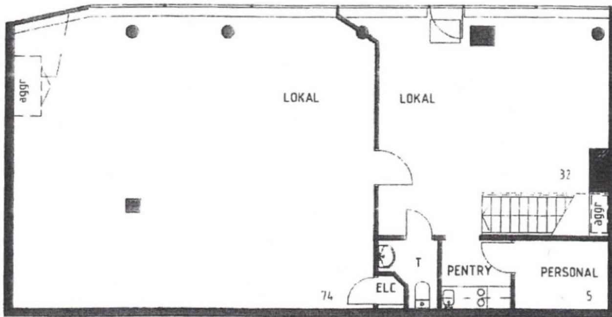
BOTTENVÅNING 122 m 2
