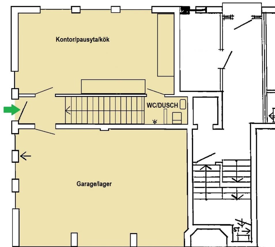
Entréplan
