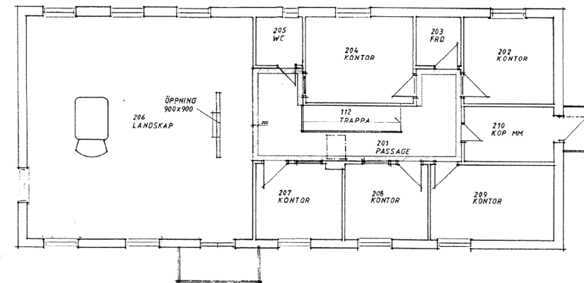
PLAN 1TR
