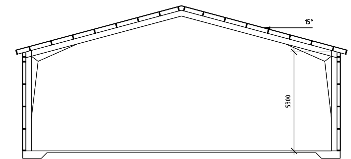
SEKTION A-A
