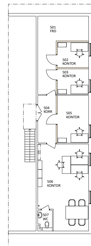
ENTRESOLPLAN LOKAL 4/5
