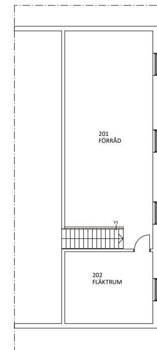
ENTRESOLPLAN LOKAL 1/2
