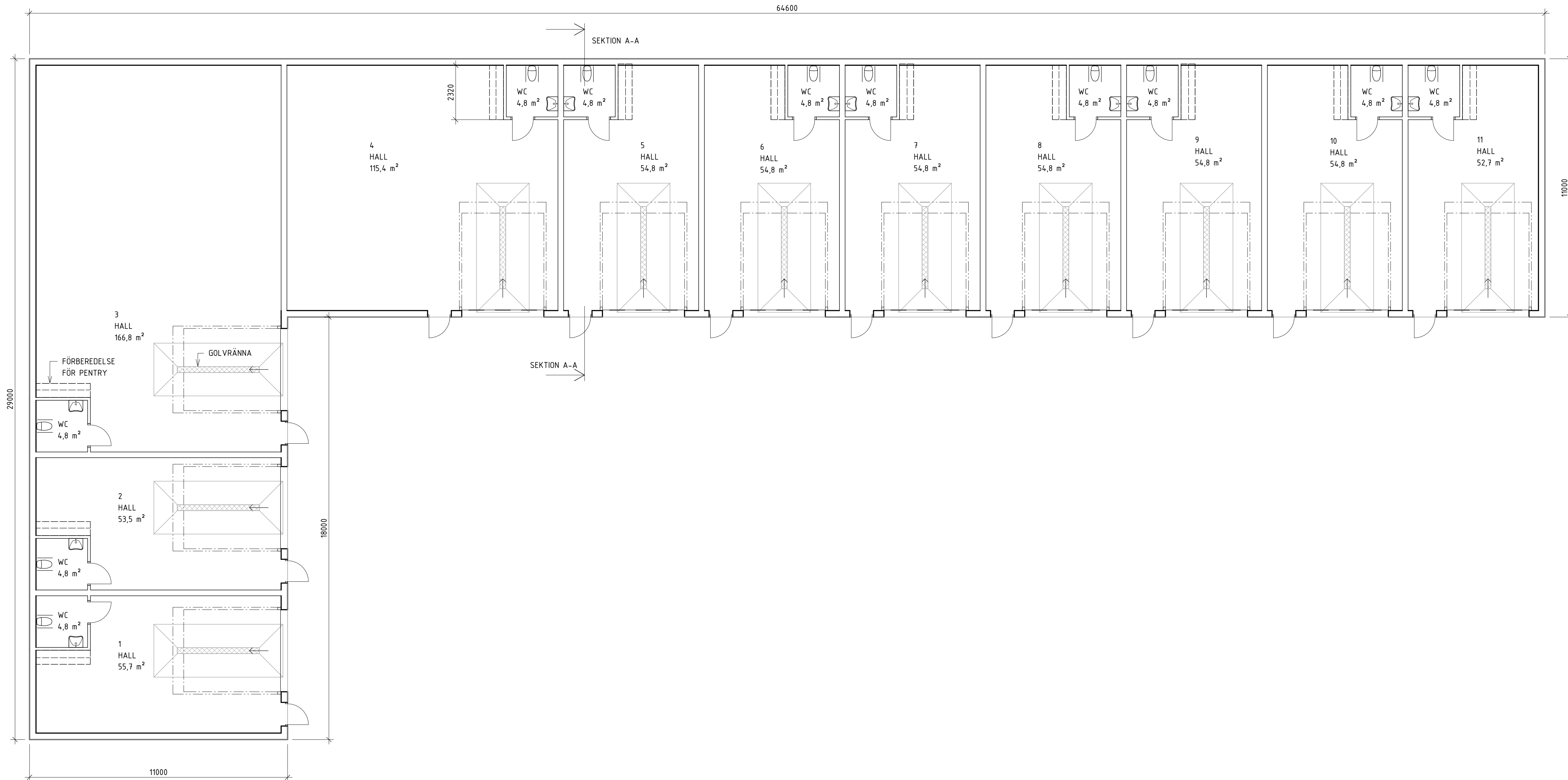
PLAN 1 1 : 100
