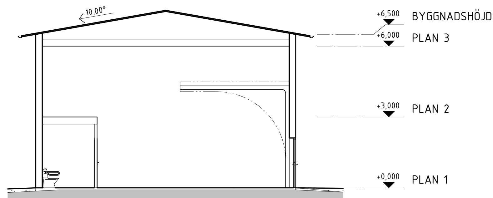
SEKTION A-A 1 : 100
