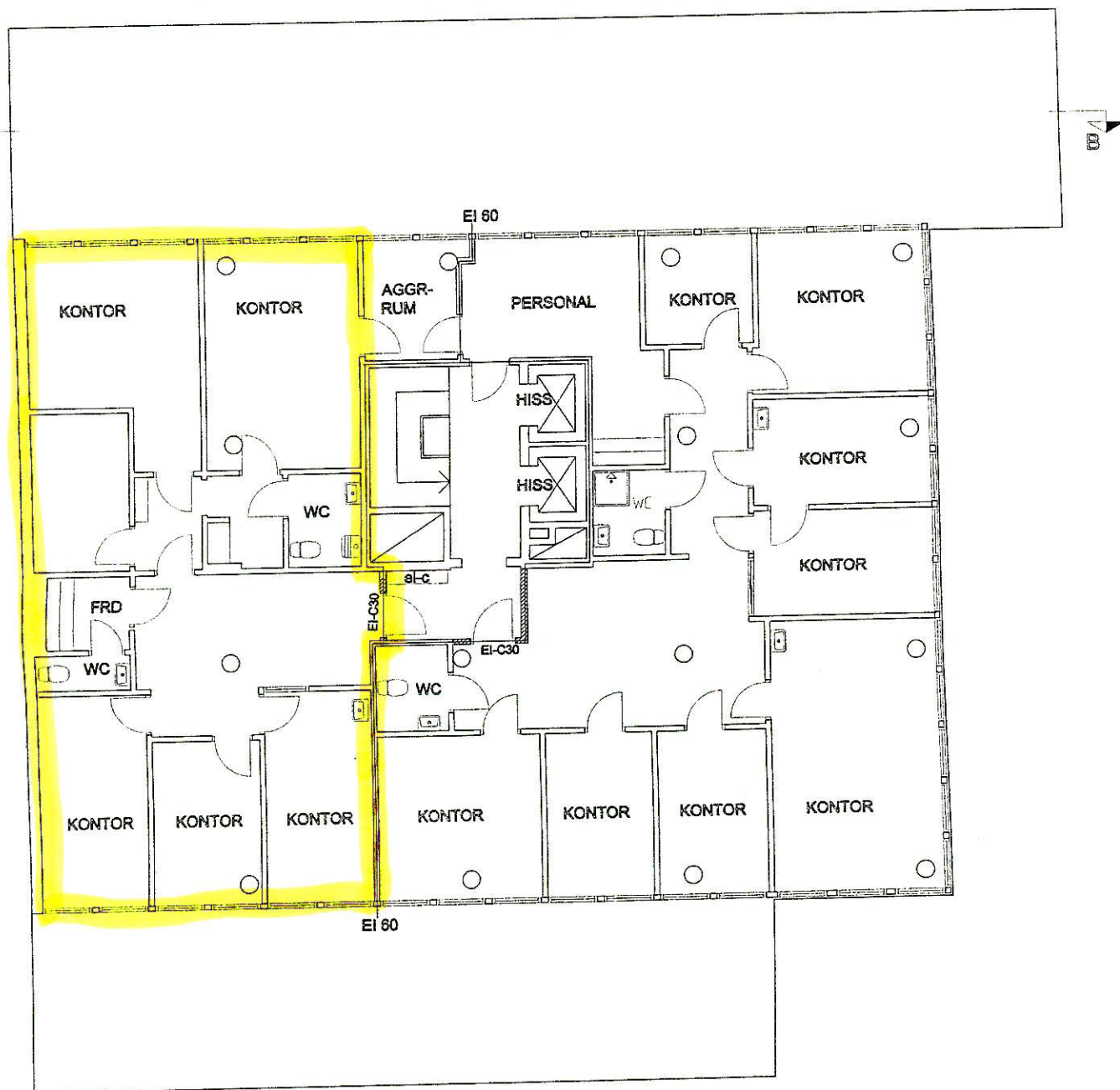
PLAN B 1:100
