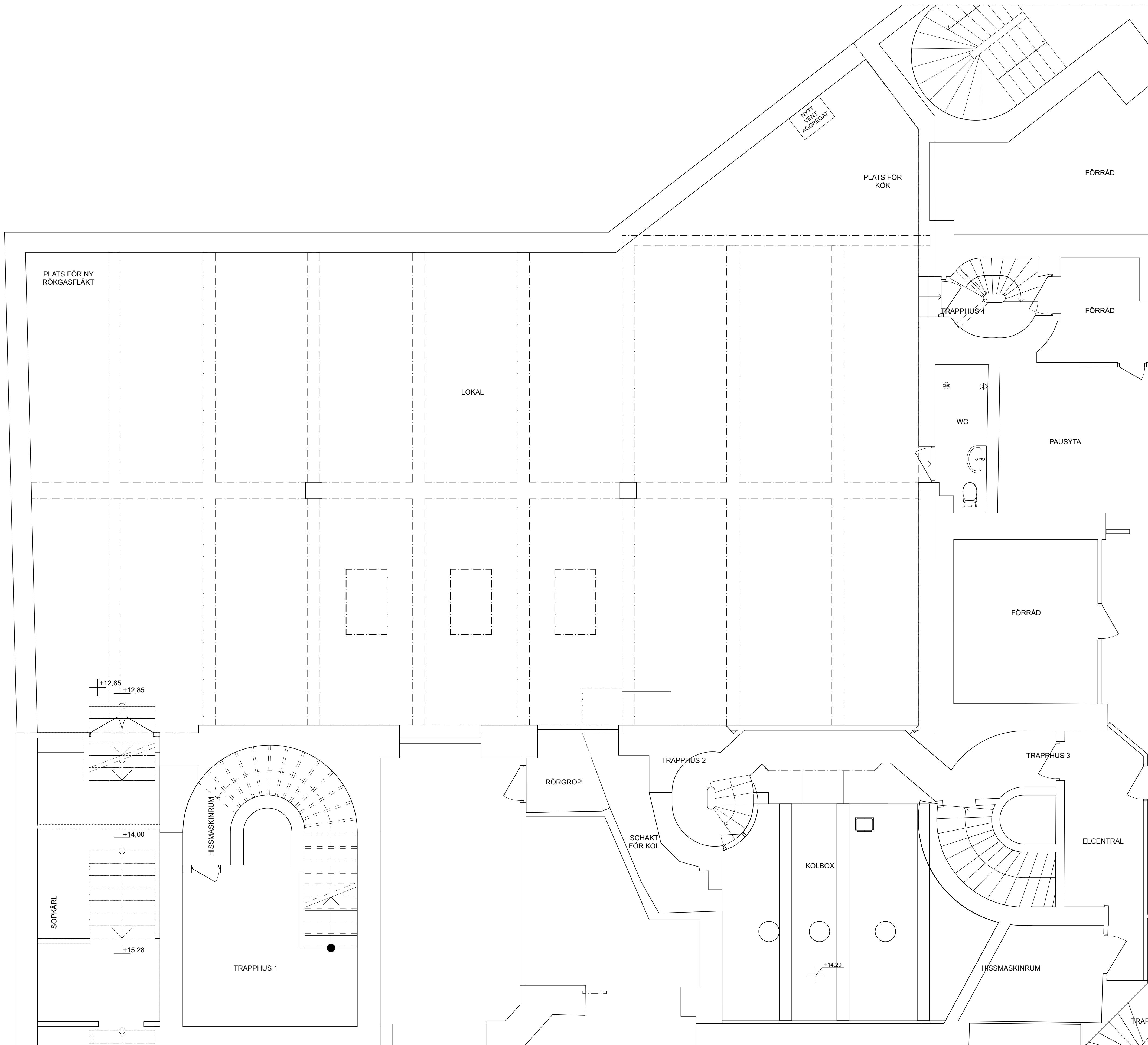
ÖVRE KÄLLARPLAN, LOKAL 1:50
