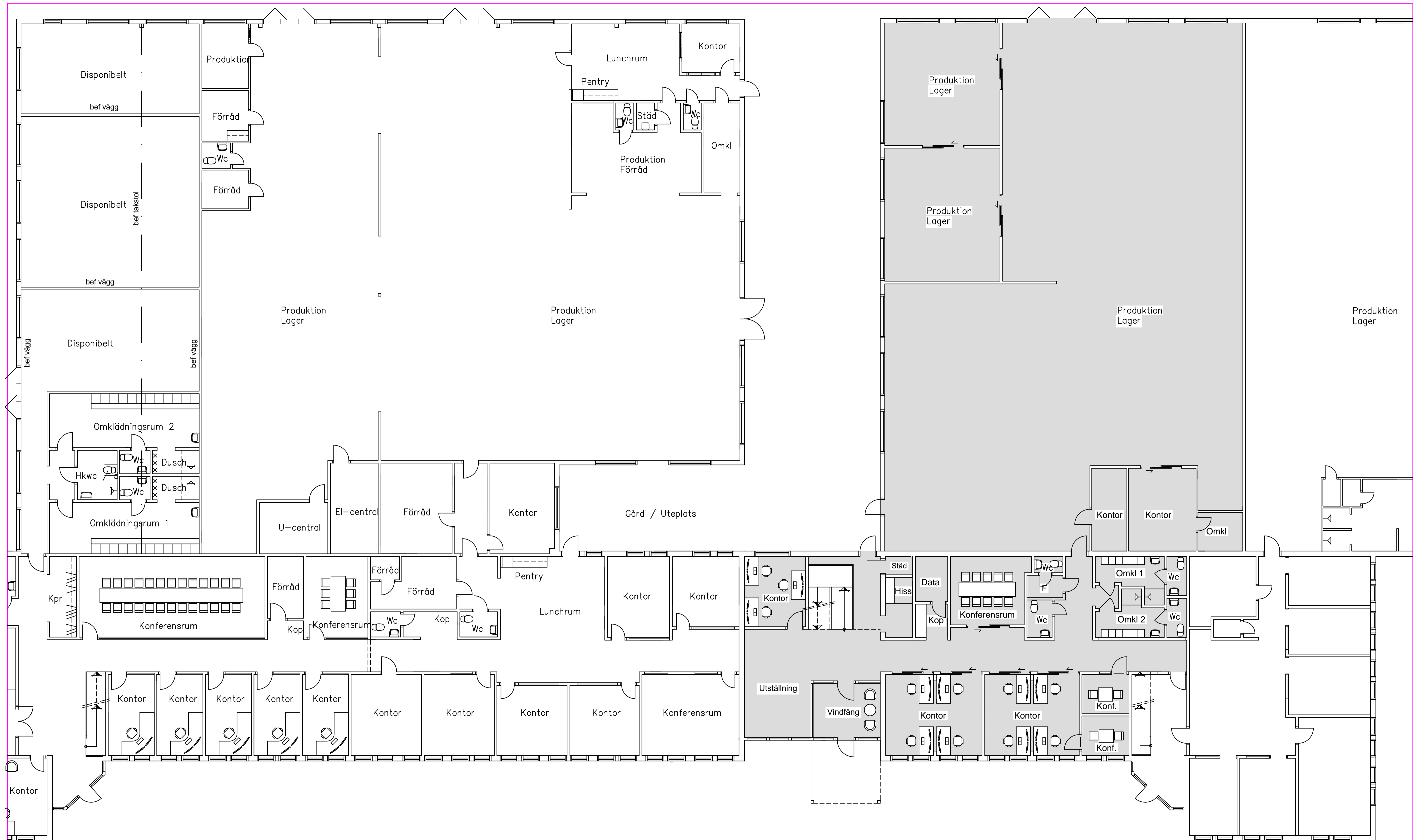
Plan bottenvåning.
