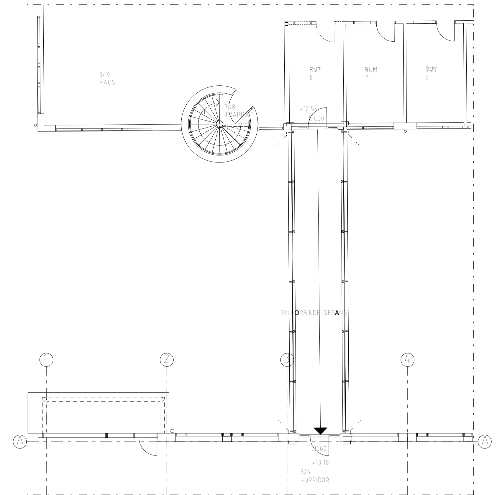
PLAN 3, GANGBRYGGA
