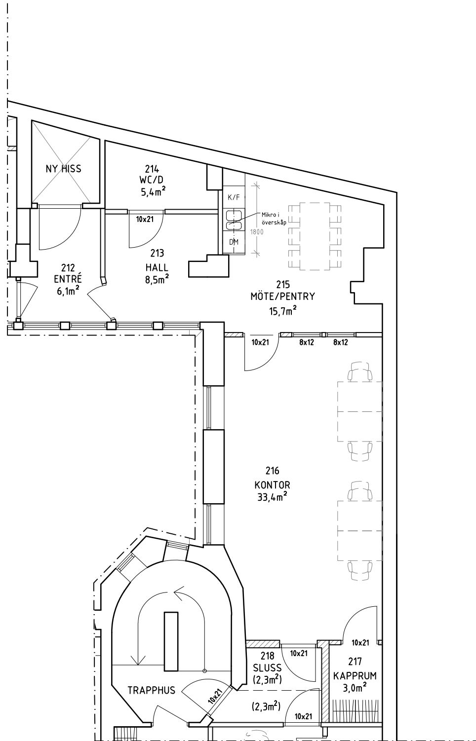
PLAN 2, DEL 2, ÖVRE 70,0m 2
